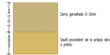
D1-PAVIMENT DE SEURETAT :SORRA
