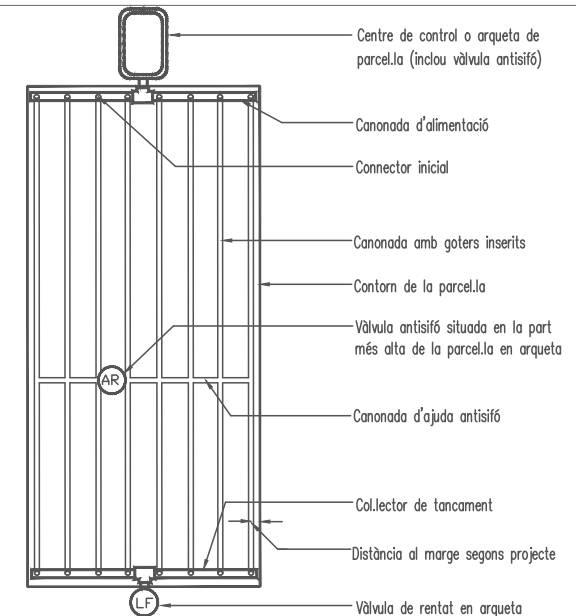
ESQUEMA VÀLVULA DE RENTAT EN ARQUETA
