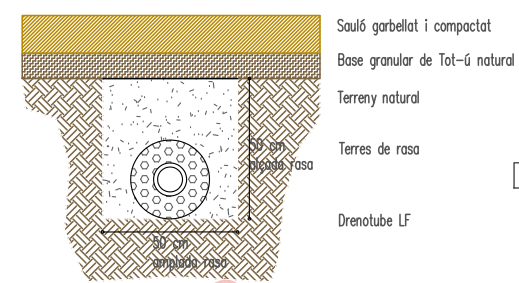
D3-DRENATGE AMB DRENOTUBE LF
