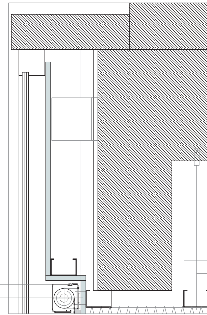
SEC. VERTICAL CAIXA JÀCENA P1
