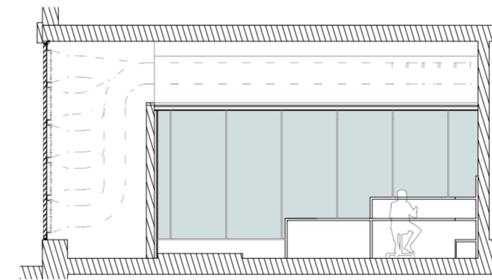
ALÇAT 4
