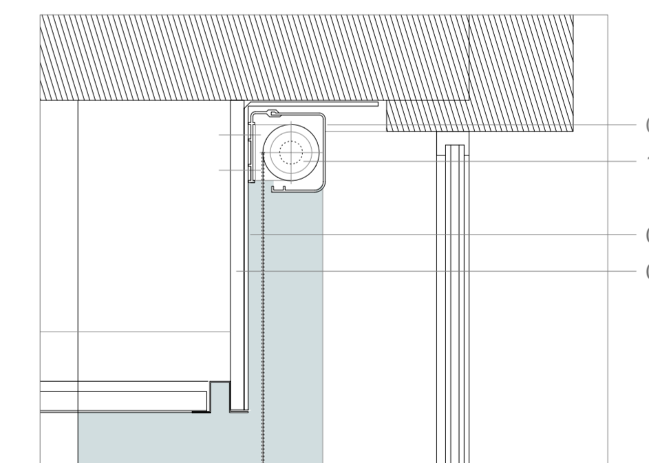
DETALL B
