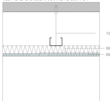
SEC. PEREPENDICULAR SOSTRE PLADUR FON
