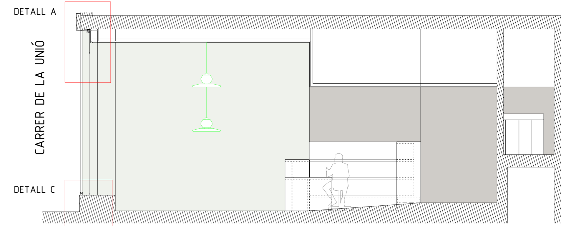
SECCIÓ 1-1
