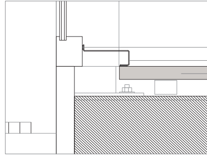
AXONIMETRIA EMPALME REMATS EN MUNTANTS
