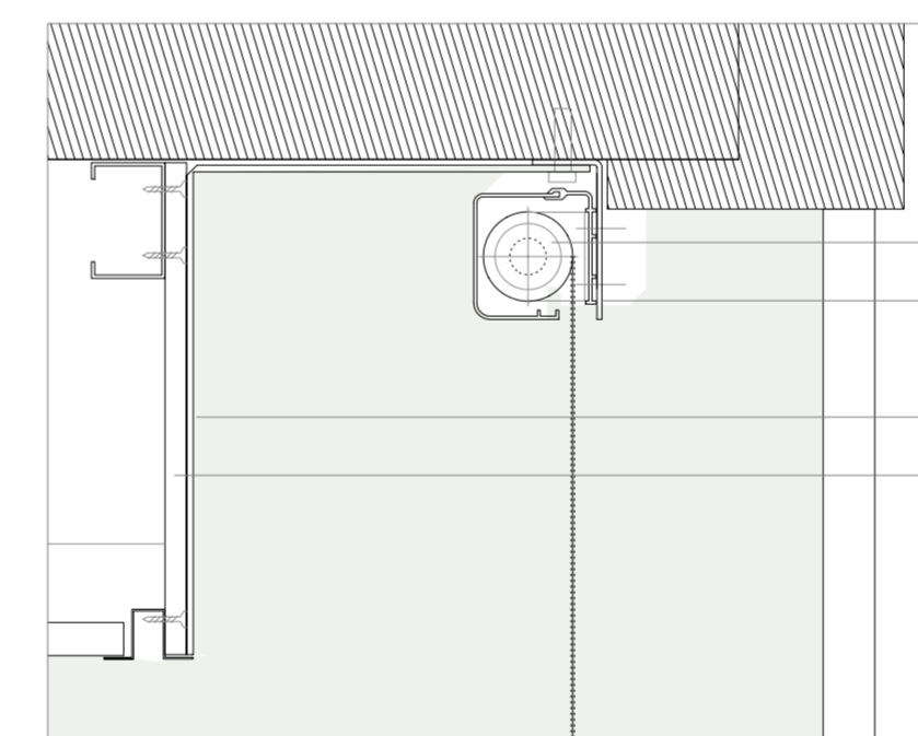
DETALL A
