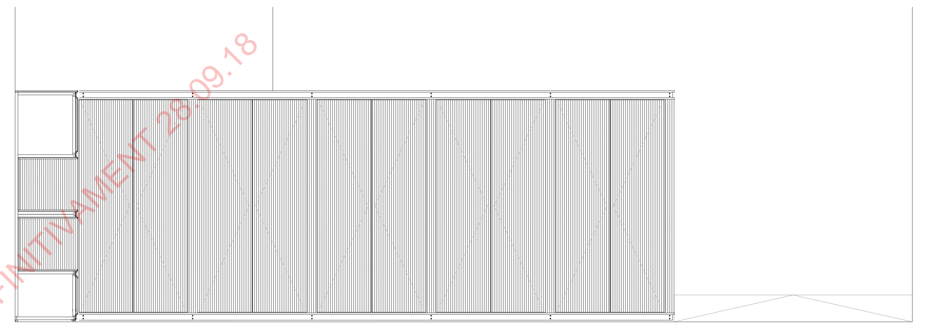
ALÇAT 2-2
