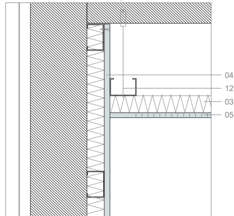
SEC. VERTICAL FINESTRA FAÇANA SUD
